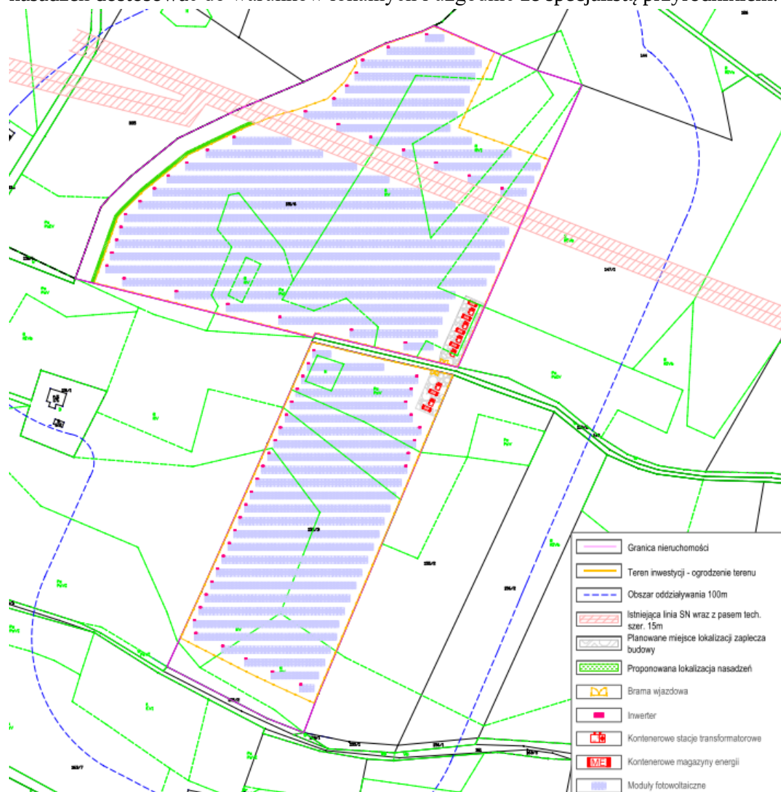
Rysunek 1. Plan zajęcia nasadzeń zieleni izolacyjnej zgodny raportem.
